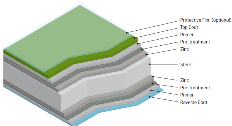
Garantiplåten/Greencoats uppbyggnad
